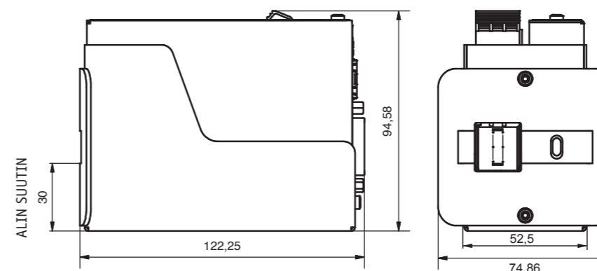
Mittapiirustus
